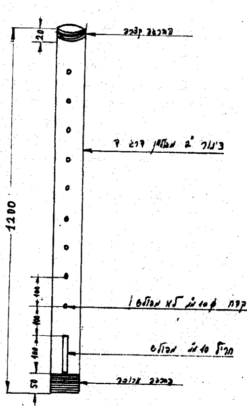
פרט א' - צינור 2"
