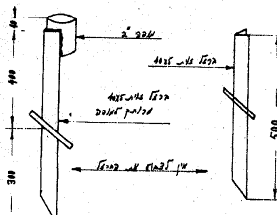
פרט ז' - יתד
